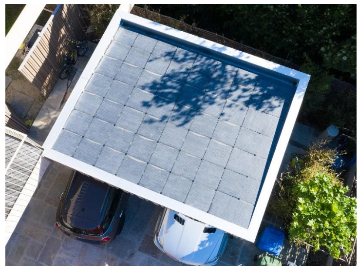
Ziegel | Tuile : Solaris Heritage, Flat 9. Oberfläche | Surface : 17 m 2 , 2.5 kWp
